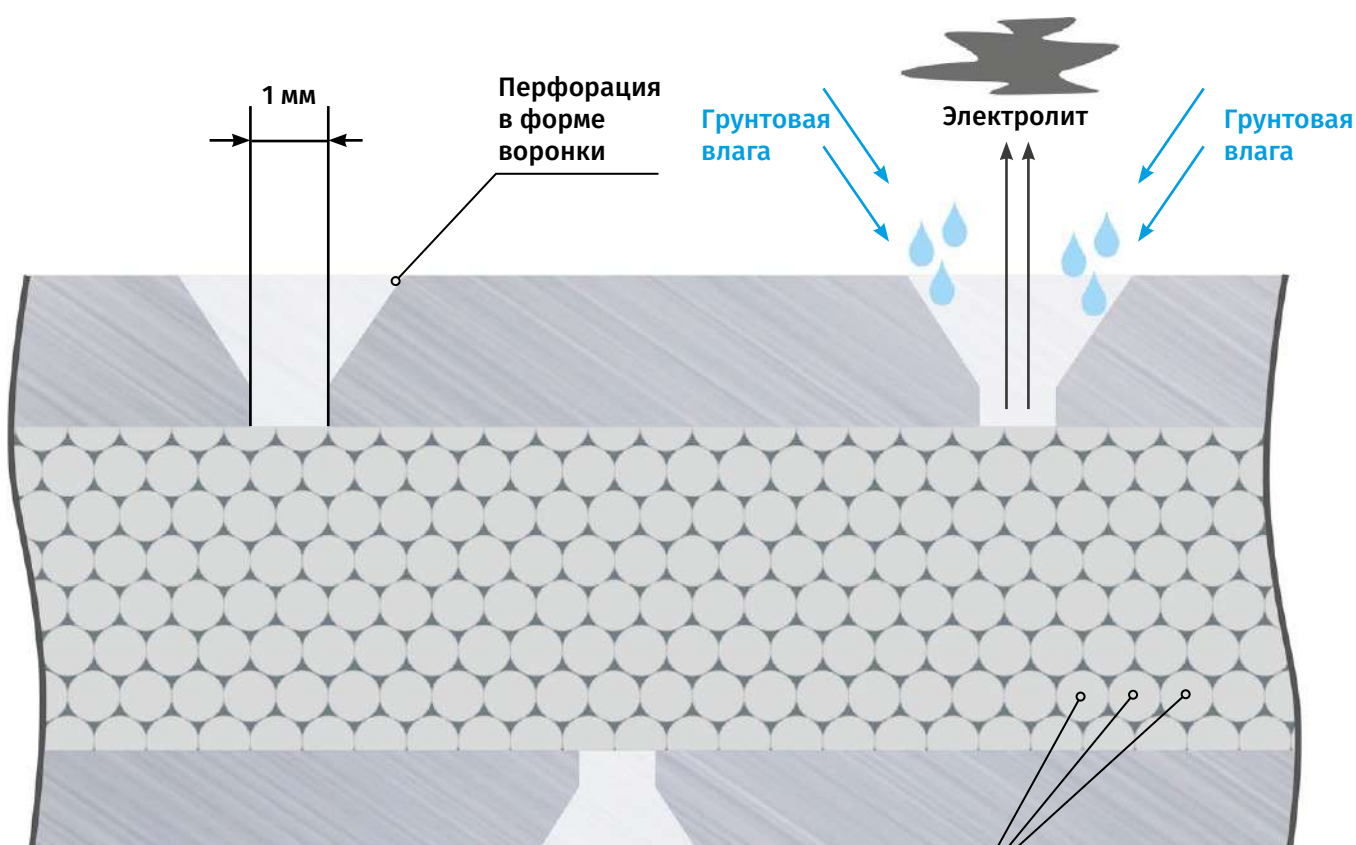
Трехкомпонентный гранулированный электролитический модуль
